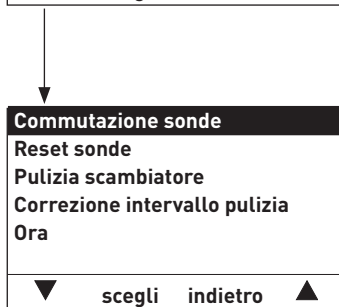
Fig. 41 Visualizzazione con sistema di alimentazione
